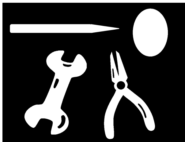
f[x,y]
